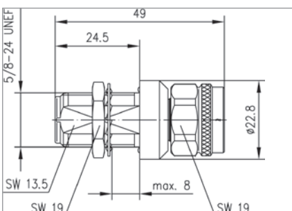
AntPro 6GHz-N (m/f)
