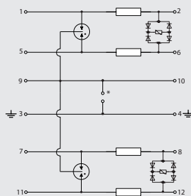
MP 2x2-170 HF ST
