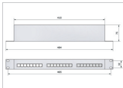
DataPro 1x8 bis 3x8RJ45-19"
