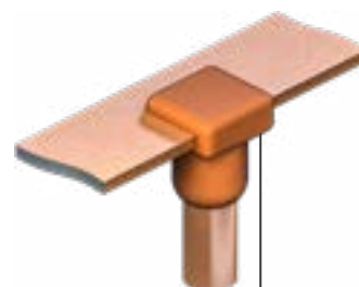
Zgrzewanie CBM Weld uziomu pomiedziowanego z bednarką pomiedziowaną
