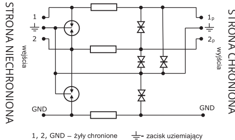
1, 2, GND – żyły chronione ⚡ – zacisk uziemiający
