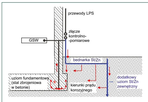
Rys. 3 Ognie elektrochemiczne powstające w wyniku połączenia uziomu fundamentowego i uziomu zewnętrznego ze stali ocynkowanej
