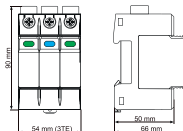
Wymiary
