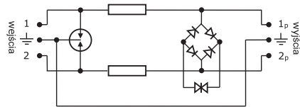
1,2 – żyły chronione — - zacisk uziemiający
